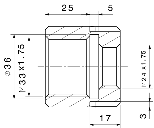
Vista A-A
